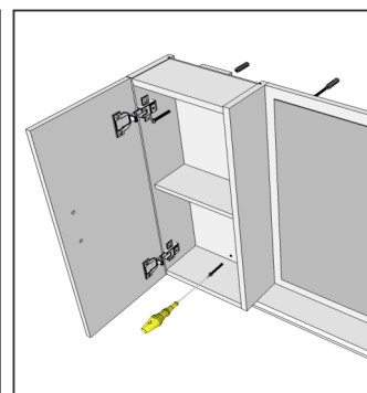
Fixação caixa espelho.
